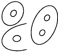
复连通区域
